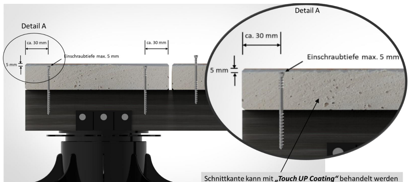
Bild 14. Die Durafix Schrauben ® müssen ca. 5 mm tief eingedreht werden und zur Längskante der Dielen ca. 30 mm Abstand haben.
