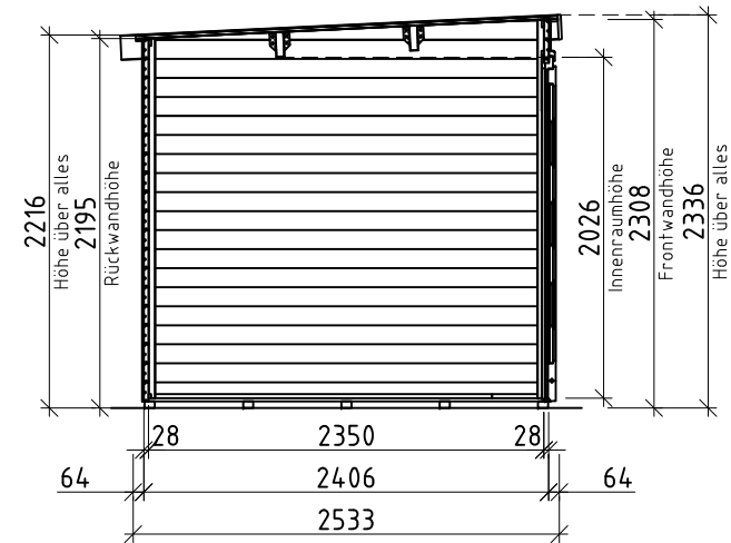
Schnitt A-A
