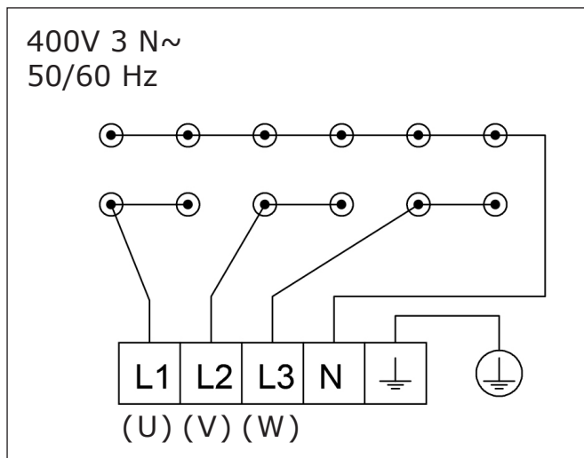
Anschlussplan für Saunaofen Durano / Durano Black mit 9,0 kW
