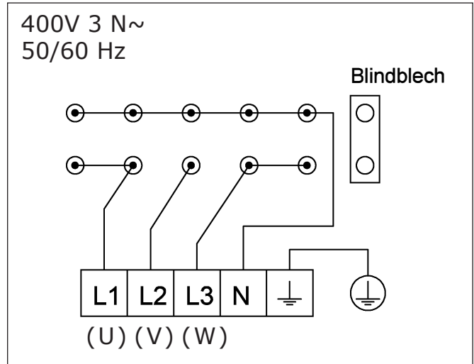
Anschlussplan für Saunaofen Durano / Durano Black mit 7,5 kW
