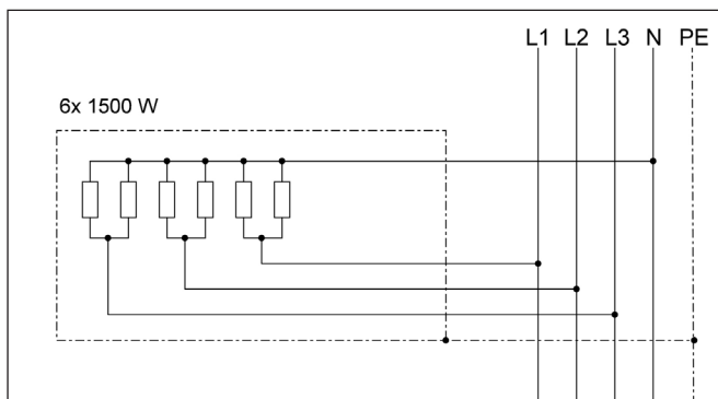
Saunaofen Durano / Durano Black mit 9,0 kW
