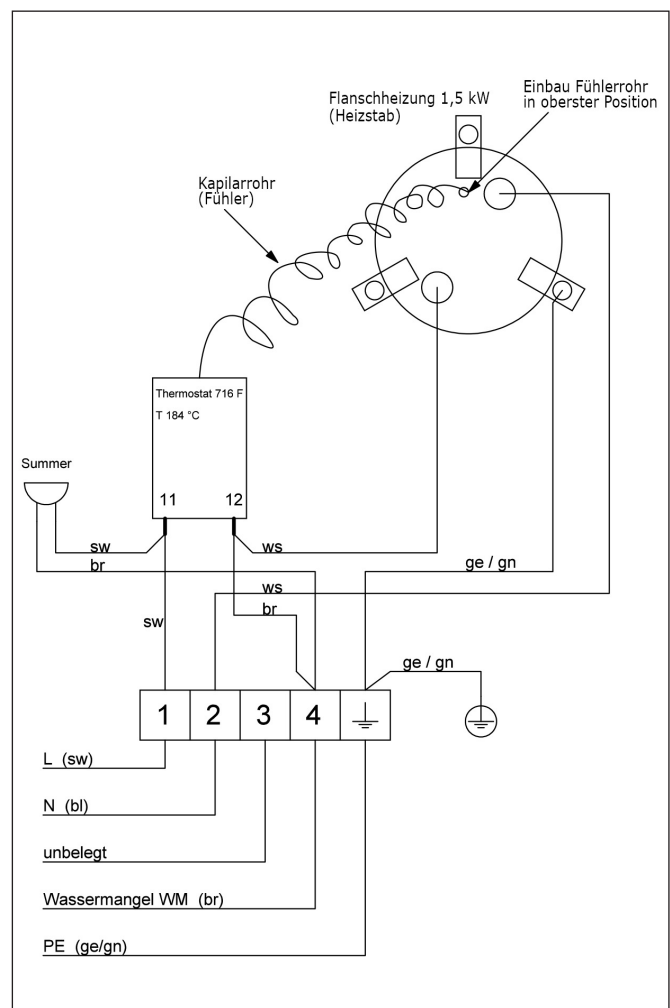
Anschlussplan für Verdampfer
