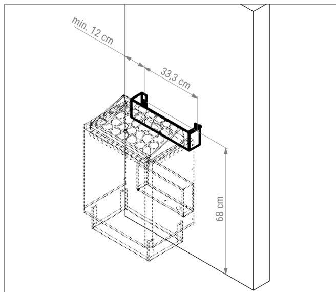
Abb. 2 - Montage Wandaufhängung
