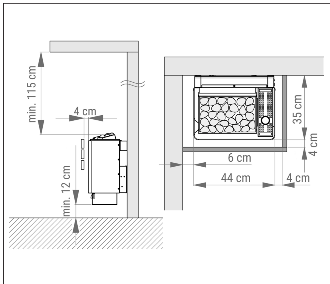
Abb. 1 - Mindestabstände
