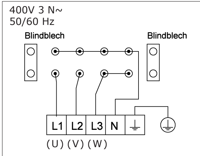
Anschlussplan für Saunaofen Durano mit 6,0 kW
