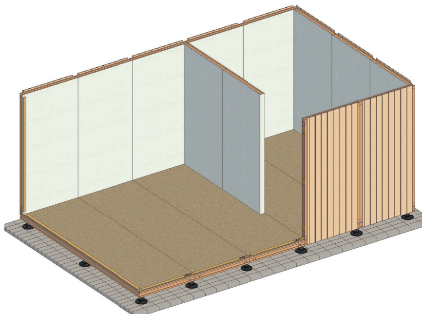
P009 Einbau der Innenwände
