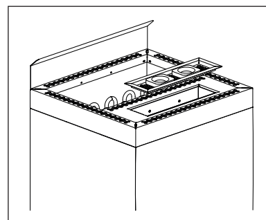
Abb. Tankabdeckung
