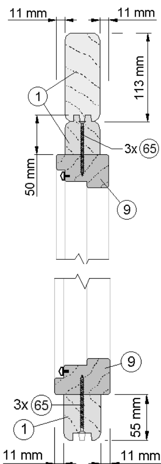
Schnitt B-B
