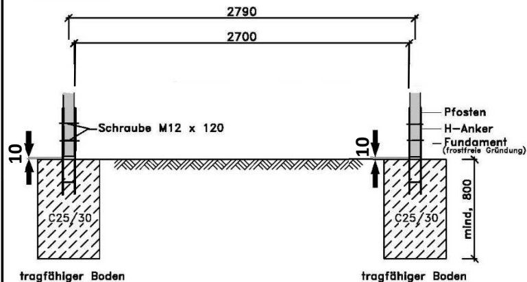
Schnitt C-C
