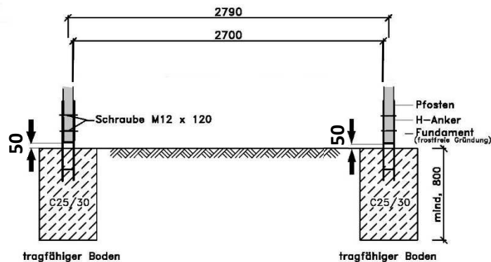
Schnitt C-C
