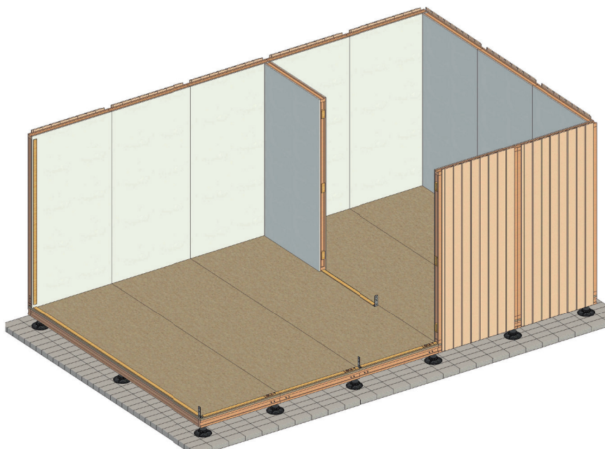
① 08 Einbau der 1. Innenwand
