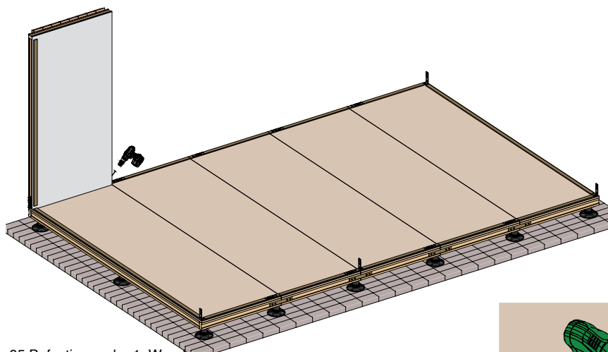
① 05 Befestigung der 1. Wand
