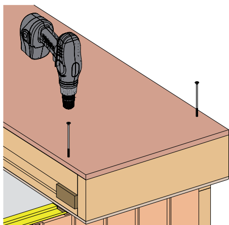
② 13 Dachbefestigung an den Wänden
