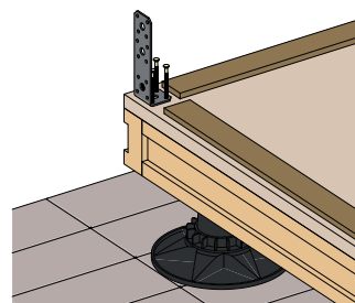
③ 04 Wandbefestigungswinkel
