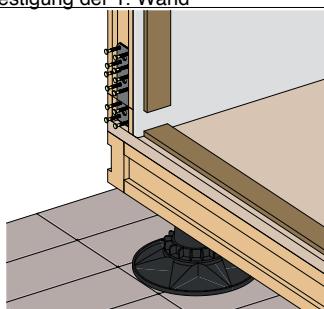
③ 05 Befestigung der 1. Wand an der Eckstütze
