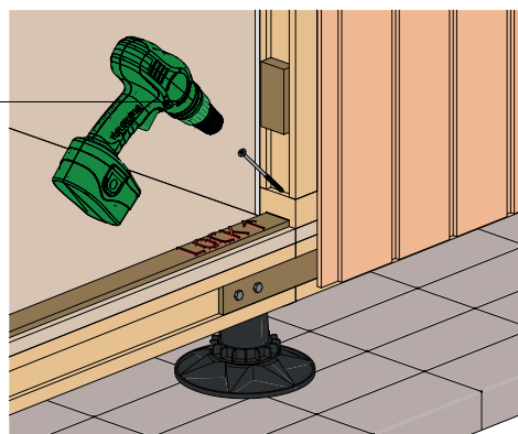
② 05 Wand-Boden-Verbindung
