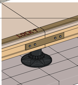
② 04 Verbindung der Böden
