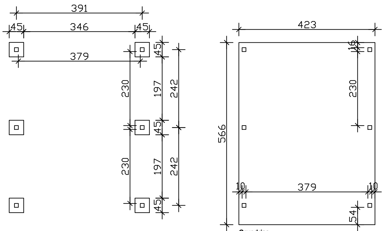
Grundriss
