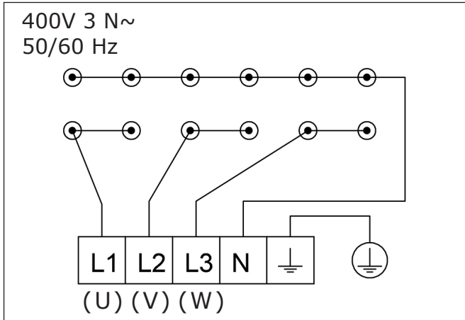
Anschlussplan für Saunaofen Ferro mit 9,0 kW / 10,5 kW
