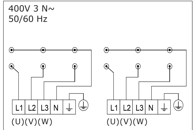
Anschlussplan für Saunaofen Ferro mit 12,0 kW (2-kreisig) mit LSG
