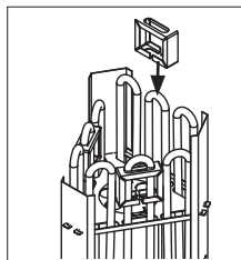
Heizelement-Abstandhalter
