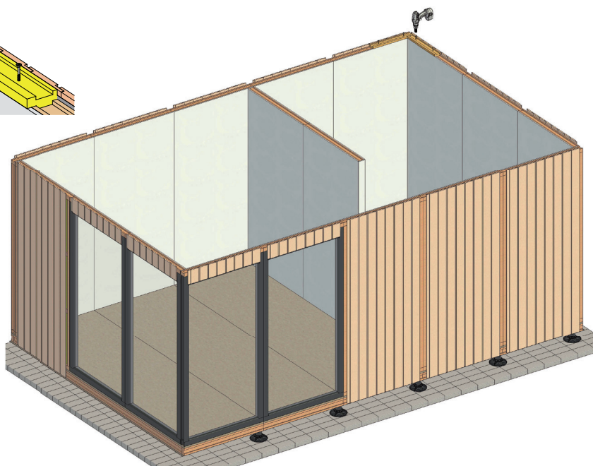
① 11 Wandgurte
