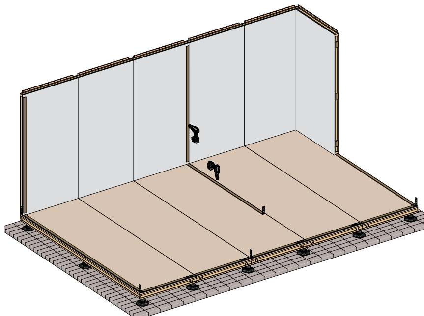
① 07 Einbau von Innenwandbefestigungen
