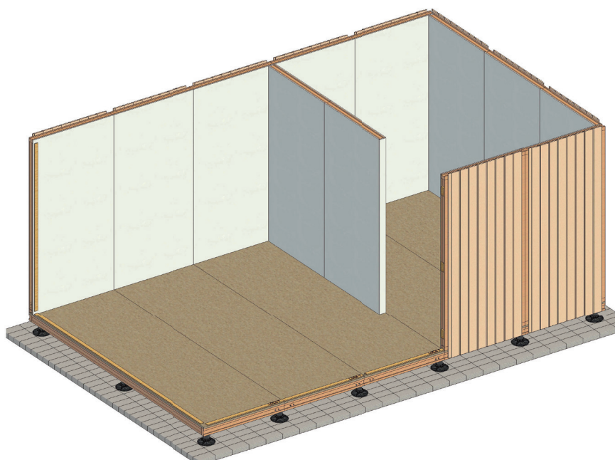
① 09 Einbau der Innenwände
