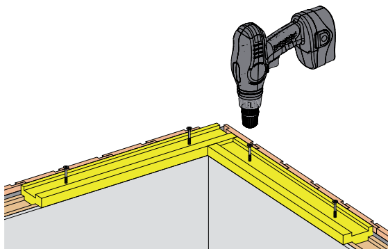
② 11 Wandgurtbefestigung
