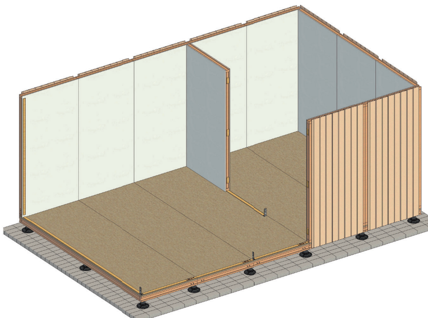
① 08 Einbau der 1. Innenwand
