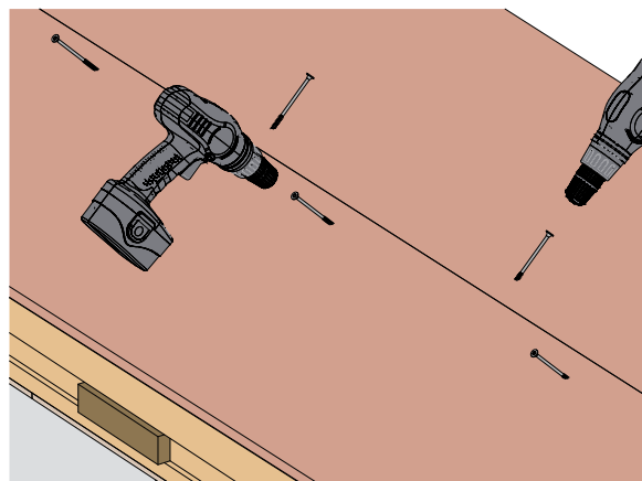
② 14 Verbindung von Dachflächen
