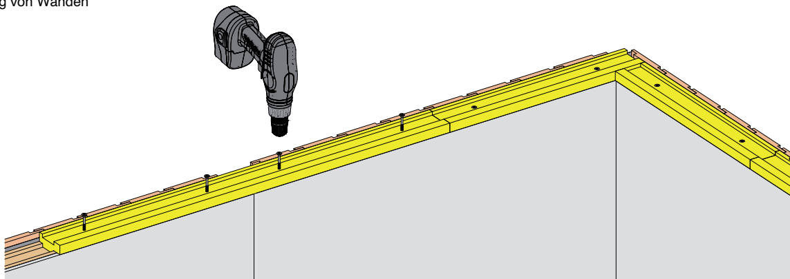
② 12 Befestigung der Wandgurte
