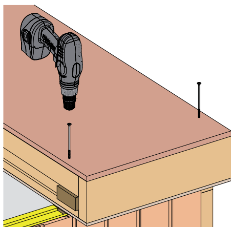
② 13 Dachbefestigung an den Wänden
