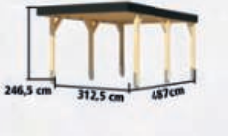
DOPPELCARPORT LEIMHOLZ 1 Seite 73
