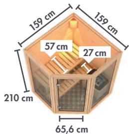
Abb. SINAI 3 mit Dachkranz, bronzierter Ganzglastür Classic und Zubehör (gegen Aufpreis)
