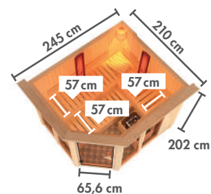
Abb. AVA mit Dachkranz, bronzierter Ganzglastür Classic
