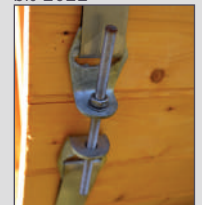
Spannring-System bis 2022
