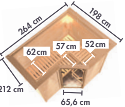
Zeichnungen und Maße mit Dachkranz
