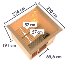
Abb. JADA, bronzierte Ganzglastür Classic, mit Zubehör (gegen Aufpreis): Kopfstütze Classic
