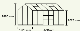
ICON PLANTHOUSE 6 · 7,3 m 2 (6' x 12')
