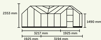
ICON GARDENHOUSE 6 · 8,6 m 2 (6' x 10')
