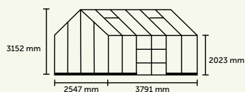
ICON PLANTHOUSE 8 · 9,7 m 2 (8' x 12')
